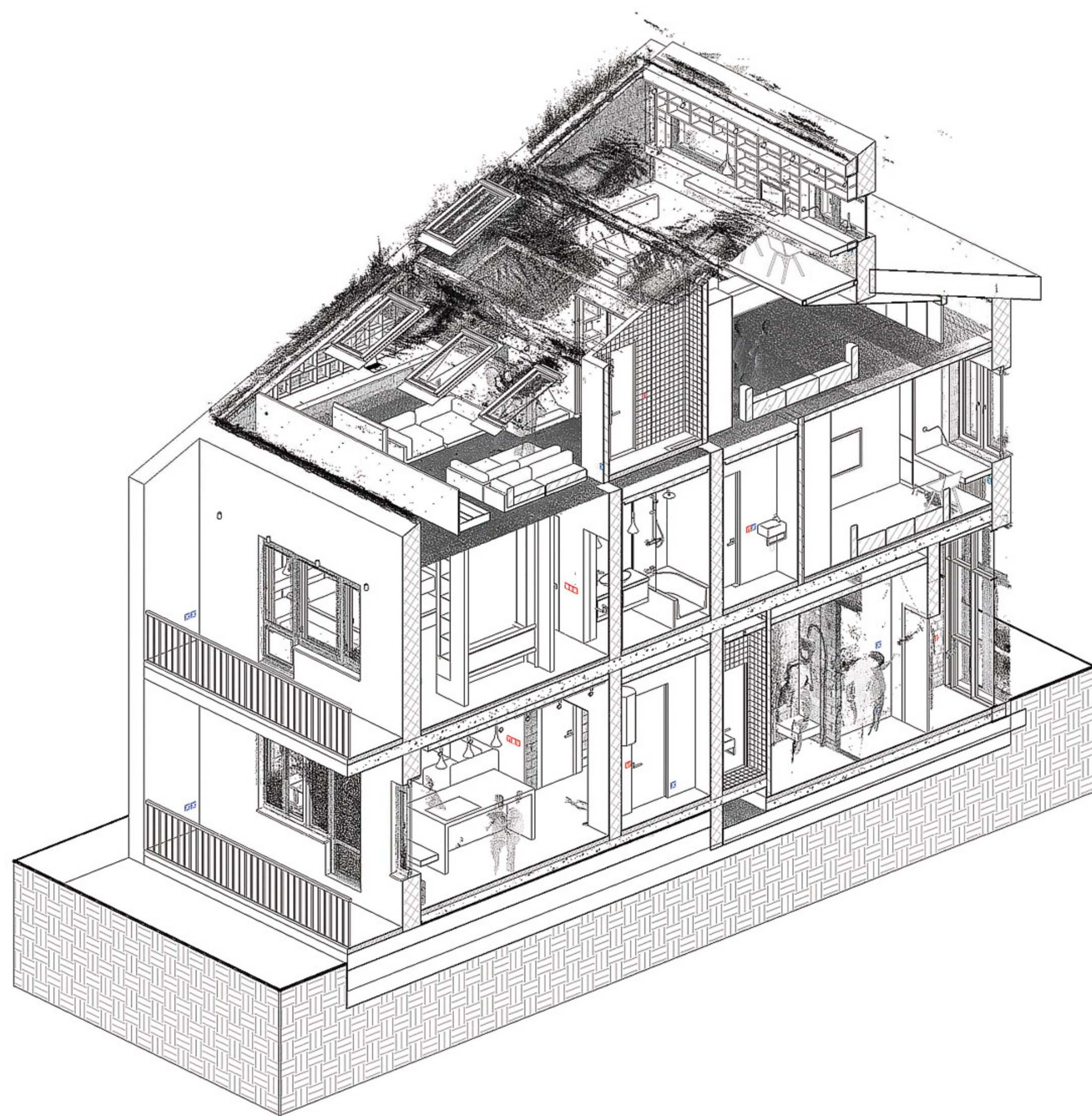
Разрез 3D модели, построенной по облаку точек и проектирование оформления интерьеров
